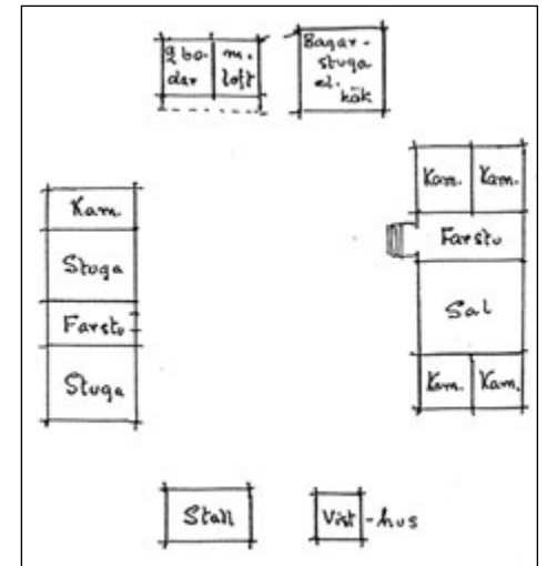
Kulhon miespihan rakennukset vuoden 1735 lähtö- ja tulokatselmuksessa annettujen tietojen mukaan. Piirustus TMK/Irja Sahlberg.
